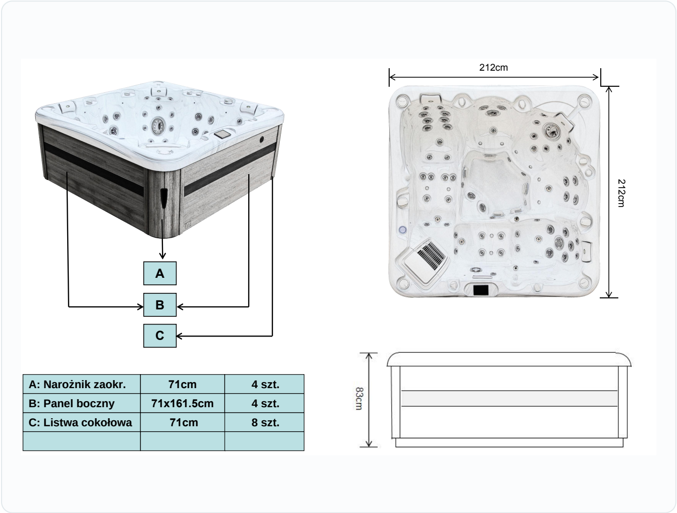
Widok 3D, rzut z góry, przekrój boczny oraz zestawienie paneli obudowy (A–C).
