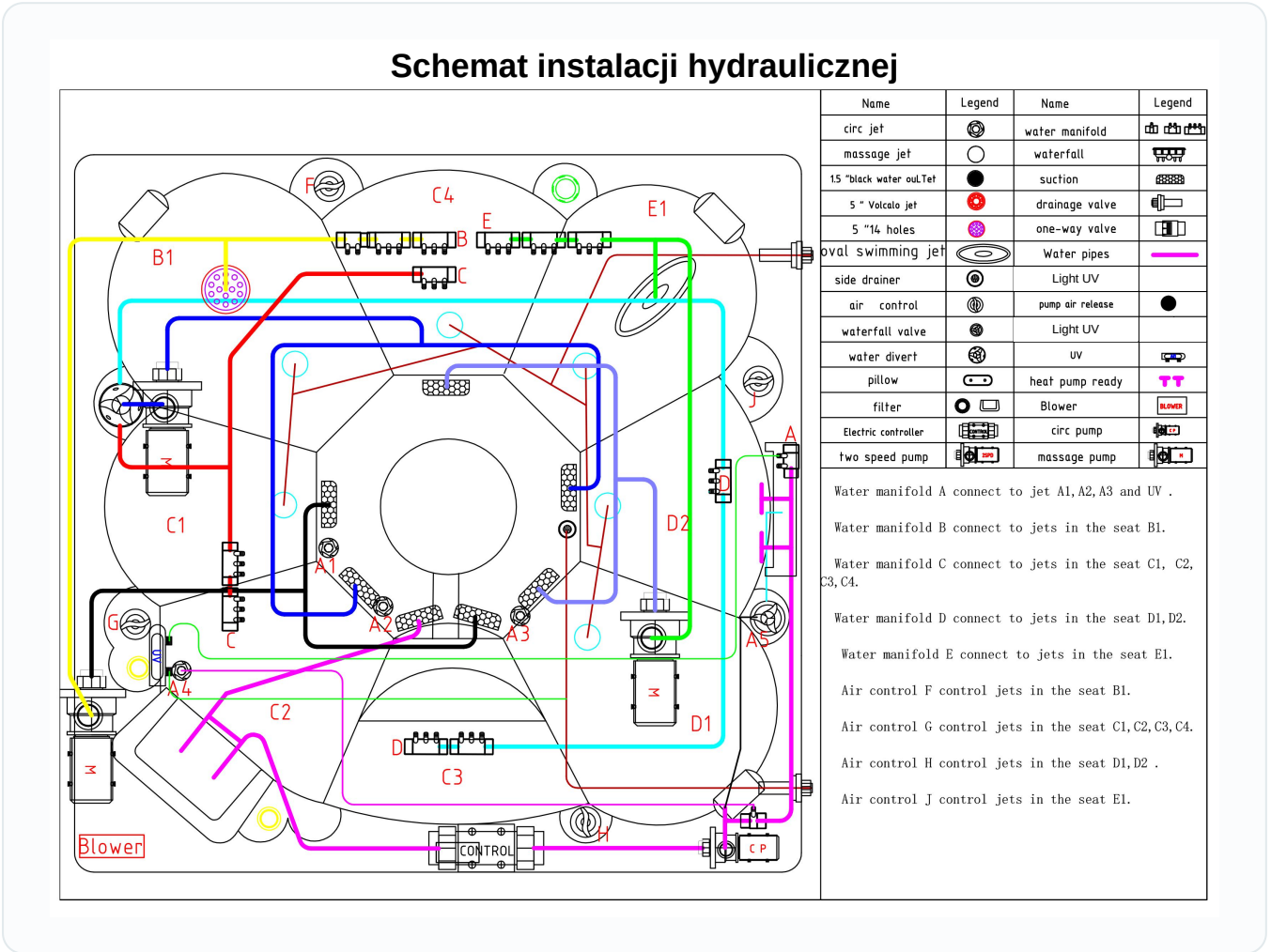
Legenda i opis połączeń kolektorów wodnych A–E wraz z funkcją sterowania powietrzem (F–H, J).
